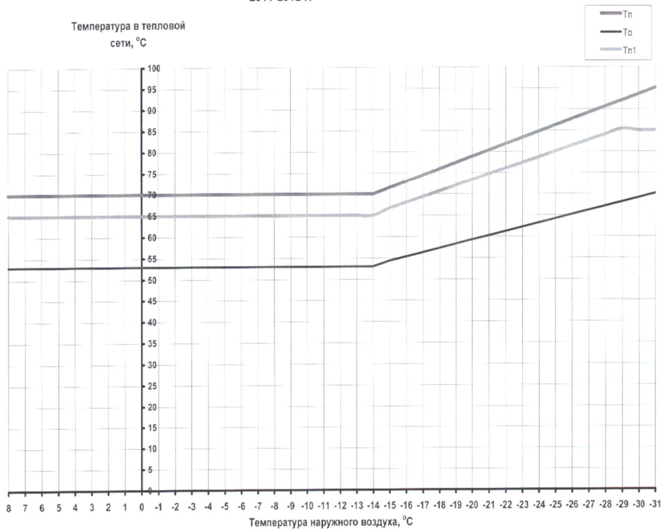
Температурный график котельной о-ва Хабарка в сезоне 2011-2012 г.
